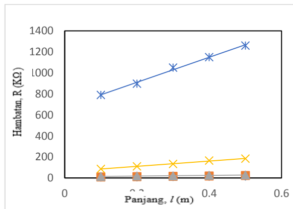
Gambar 1. Grafik antara hubungan antara panjang selang, l (m) dengan hambatan, R (K. \Omega )
