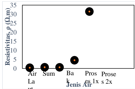
Gambar 2. Grafik hubungan jenis air, dengan resistivitas, \rho ( \Omega.m )
