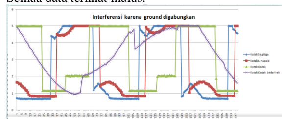
Gambar 5. Sinyal terinterferensi
