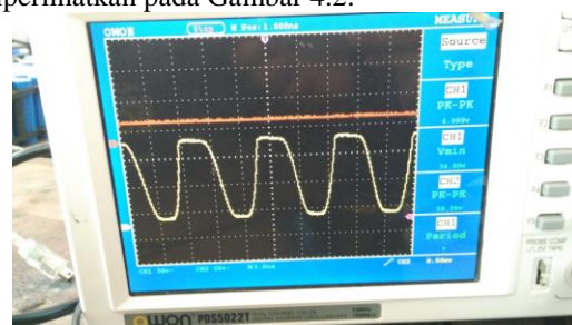
Gambar 2.2 Bentuk gelombang pada kaki transistor (emittor kolektor)
