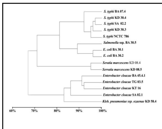
Gambar 1. Dendrogram yang menunjukkan hubungan similaritas antara 15 strain bakteri batang gram negatif hasil isolasi dari sampel darah Widal positif pada pasien gejala klinis demam tifoid asal Kota Semarang yang didasarkan atas analisis Simple Matching Coefficient (SSM) dan algoritme UPGMA.
