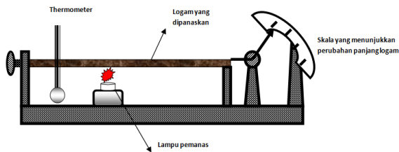
Gambar 2. Alat Muai Panjang
