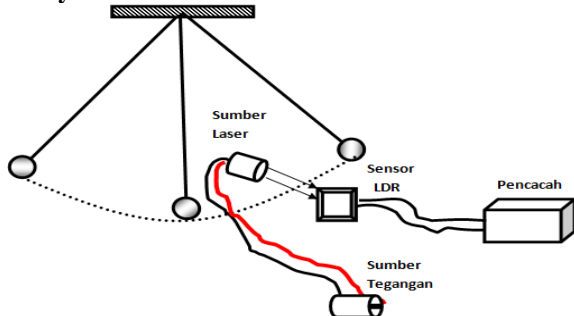
Gambar 3. Ayunan Matematis
