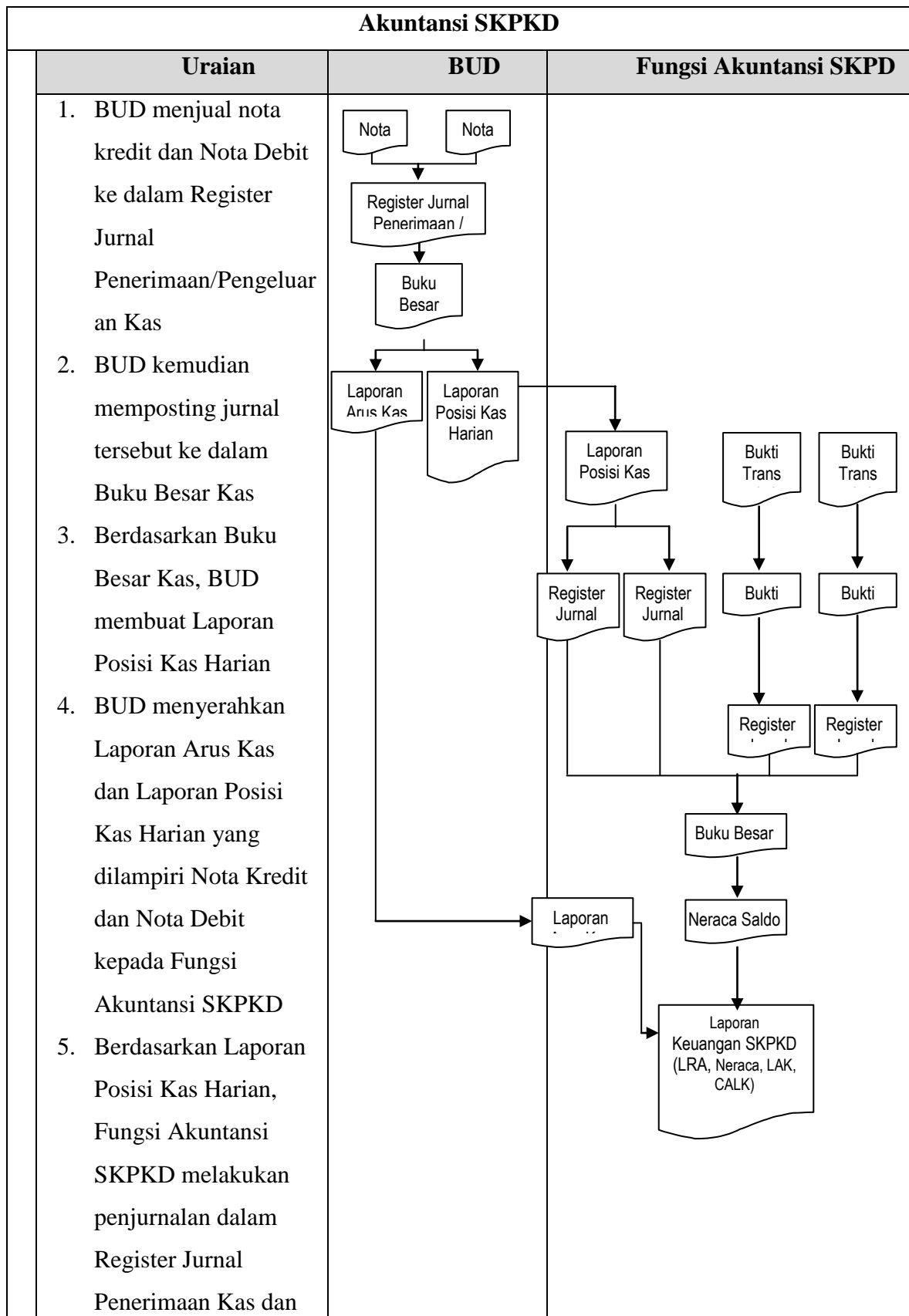
Gambar 9. Akuntansi SKPKD-2
